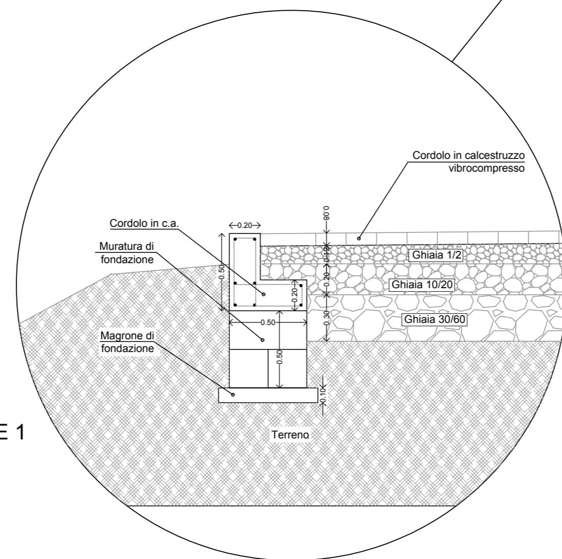
SEZIONE A-A
